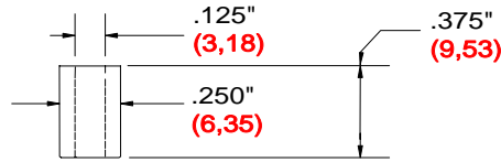
TX-375-125 DRB DRILL BUSHING
