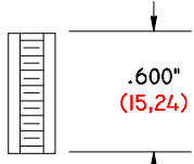
TX-600-250/6-32 DS .600" (15,24) LONG .250" (6,35) Ø O. D. 6-32 THREAD DELRIN SPACER
