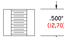
TX-500-500/8-32 DS .500" (12,70) LONG .500" (12,70) Ø O. D. 8-32 THREAD DELRIN SPACER
